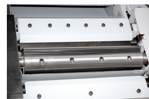
Albero di spianatura da Ø 70 mm con 3 ferri 310 x 25 x 3 mm
