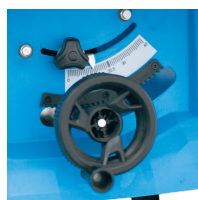
Lame réglable en hauteur par une manivelle.
