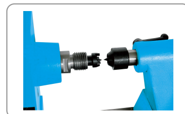
Allineamento punte cm2 e mandrino di trasmissione filettato m33 x 3,5 mm
