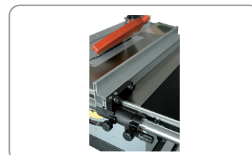
Guida di rifinitura con regolazione micrometrica
