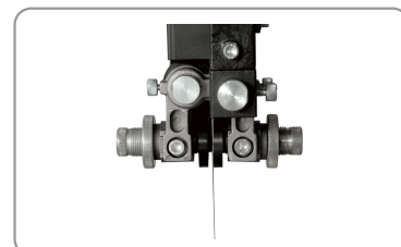
Guida lama superiore e lama inferiore a rotelle
