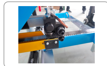
Guida e protezione della lama regolabili
