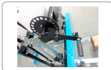
Manovella per la regolazione dell'altezza di taglio
