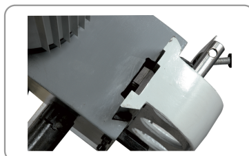
Scorrimento testa su coda di rondine
