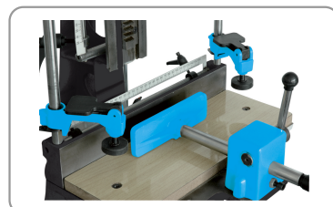
2 pressori verticali a serraggio rapido e 1 pressore orizzontale scorrevole
