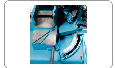
Arco orientable de 0° a 60° a la izquierda para los cortes angulados
