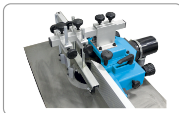
Guía de tupí con prensos horizontal y vertical
