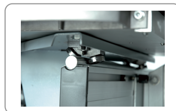
Carro de ranuración con deslizamiento sobre rodamiento de bolas
