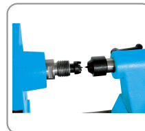
Alineación de los puntos cm2 y broca de accionamiento roscada m33 x 3,5 mm
