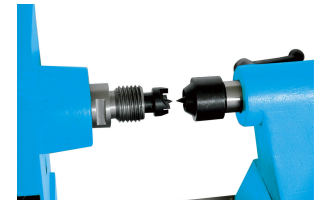
Cabezal de acero fundido, broca de alimentación m33 x 3,5 mm
