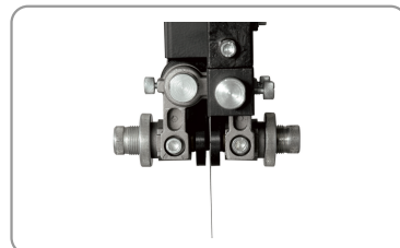
Guía de hoja superior e inferior con rodillos
