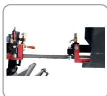
Guía de la hoja ajustable y muy precisa mediante rodamientos de 8 puntos
