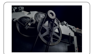
Rodillos accionados por cadena, accionamiento por motor de doble correa
