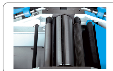
Rodillos de arrastre Ø 40 mm para alimentar la pieza, huso de 4 fierros de 95 mm
