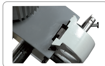
Deslizamiento del cabezal en cola de milano
