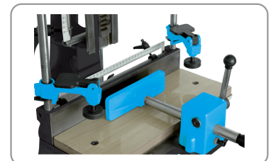
2 prensos verticales de apriete rápido y 1 prensor horizontal deslizante
