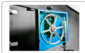
Volantes de aluminio fundido equilibrados y contactores de seguridad
