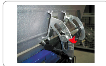
Guía de perfil de aluminio con inclinación de 45°
