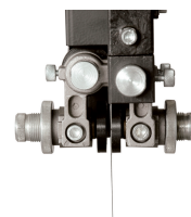
Guía de hoja superior e inferior con rodillos
