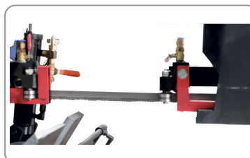
Guía de la hoja ajustable y muy precisa mediante rodamientos de 8 puntos
