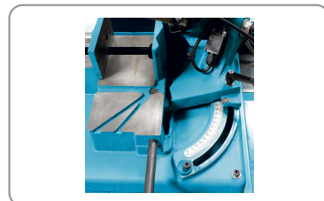
Arco orientable de 0° a 60° a la izquierda para los cortes angulados
