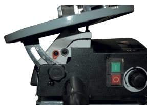
Mesa de aluminio fundido con inclinación de 45°
