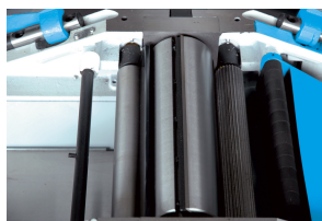
Rodillos de arrastre Ø 40 mm para alimentar la pieza, huso de 4 hierros de 95 mm
