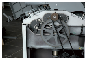
Accionamiento mediante cadena, accionamiento del motor con doble correa
