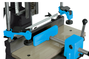
2 prensos verticales de apriete rápido y 1 prensor horizontal deslizante
