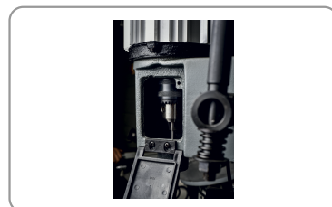
Sistema de mandril para fijación de la fresa
