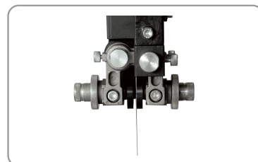
Guía de hoja superior e inferior con rodillos
