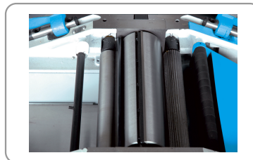
Rodillos de arrastre Ø 40 mm para alimentar la pieza, huso de 4 hierros de 95 mm
