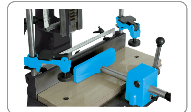
2 prensos verticales de apriete rápido y 1 prensor horizontal deslizante
