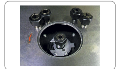
5 pinzas de apriete (6 - 6,35 - 8 - 12 - 12,7 mm)
