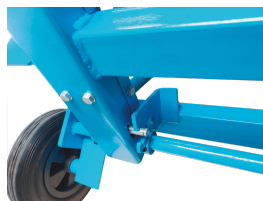
Interverrouillage du chariot de coupe et du protecteur supérieur.
