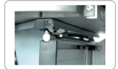
Chariot de tenonnage avec coulissement sur roulements à billes
