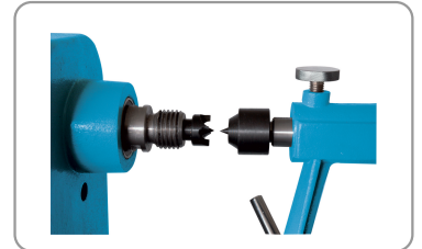
Broche entraînement cm2 filetée m33 x 3,5 mm
