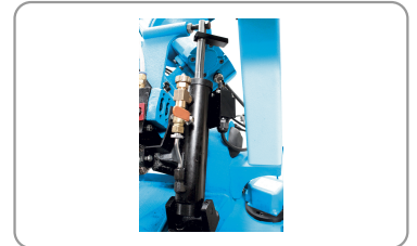
Descente de l'archet par vérin hydraulique avec débit réglable
