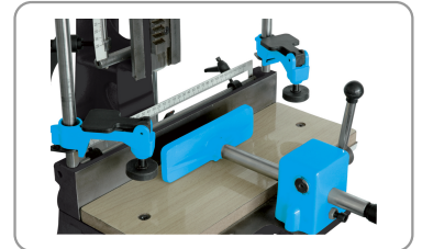
2 presseurs verticaux à serrage rapide et 1 presseur horizontal coulissant
