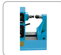
Broche dentrainement cm2 filetée m33 x 3,5 mm
