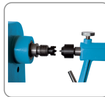
Broche entraînement cm2 fileté m33 x 3,5 mm
