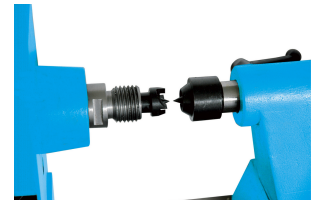
Tête en fonte d'acier, broche entraînement m33 x 3,5 mm
