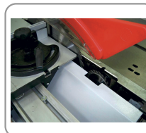
Lame Ø 315 mm, inclinable à 45° et inciseur de 100 mm
