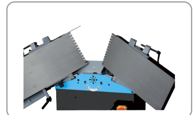
Ouverture papillon
