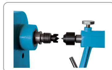
Broche d'entraînement cm2 filetée m33 x 3,5 mm
