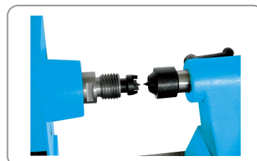
Alignement des pointes cm2 et broche d'entraînement filetée m33 x 3,5 mm
