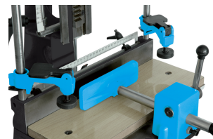
2 presseurs verticaux à serrage rapide et 1 presseur horizontal coulissant
