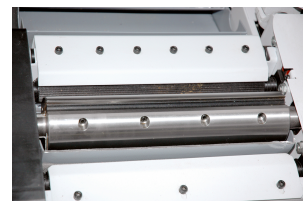
Arbre de dégauchissage de Ø 70 mm avec 3 fers 310 x 25 x 3 mm
