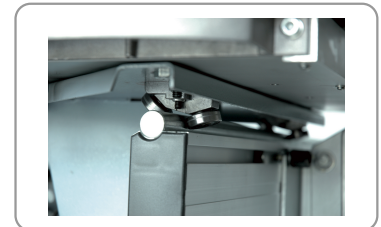
Chariot de tenonnage avec coulissement sur roulements à billes
