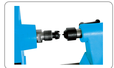
Alignement des pointes cm2 et broche dentrainement fileté m33 x 3,5 mm
