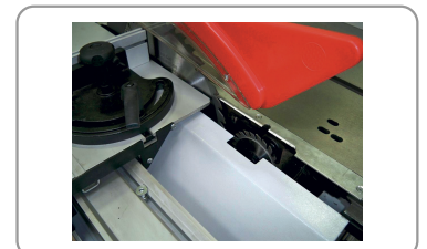
Lame Ø 315 mm, inclinable à 45° et inciseur de 100 mm
