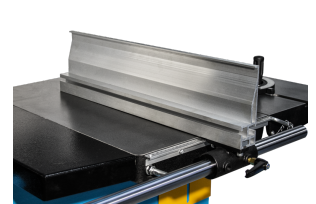
Guide de refente offrant 2 surfaces d'appui
