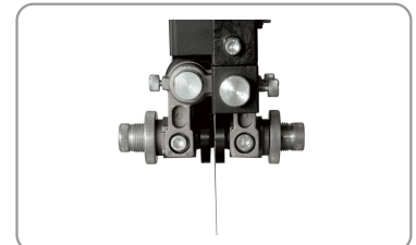
Guide de lame supérieur et inférieur à galets
