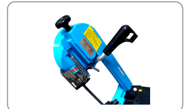
Poignée de réglage de la tension de la lame
