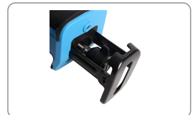
Collet à serrage rapide et sabot orientable.
